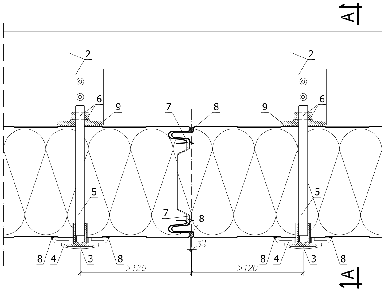
Przekrój A-A
