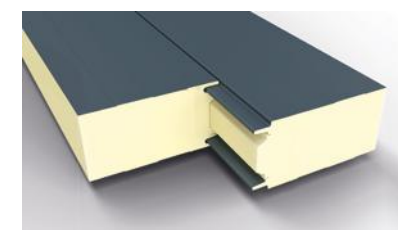
Schloss für GS insPIRe® CH Kühlplatte
