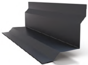
Innenecke zum Verdecken von Verbindern
