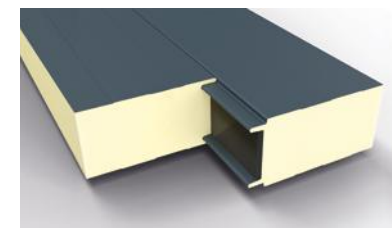
Standardschloss für GS insPIRe® S Wandplatten
