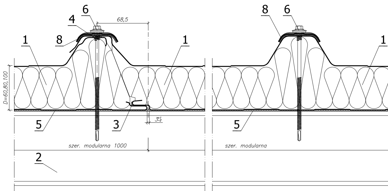
Przekrój A-A
