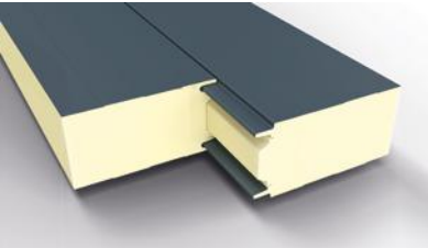
Zamek dla płyty chłodniczej GS insPIRe® CH
