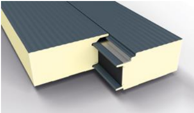
Zamek ukryty dla płyty ściennej GS insPIRe® U
